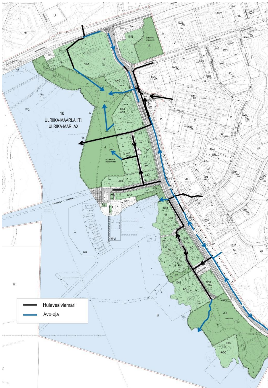
Hulevesien johtamisperiaatteet.
